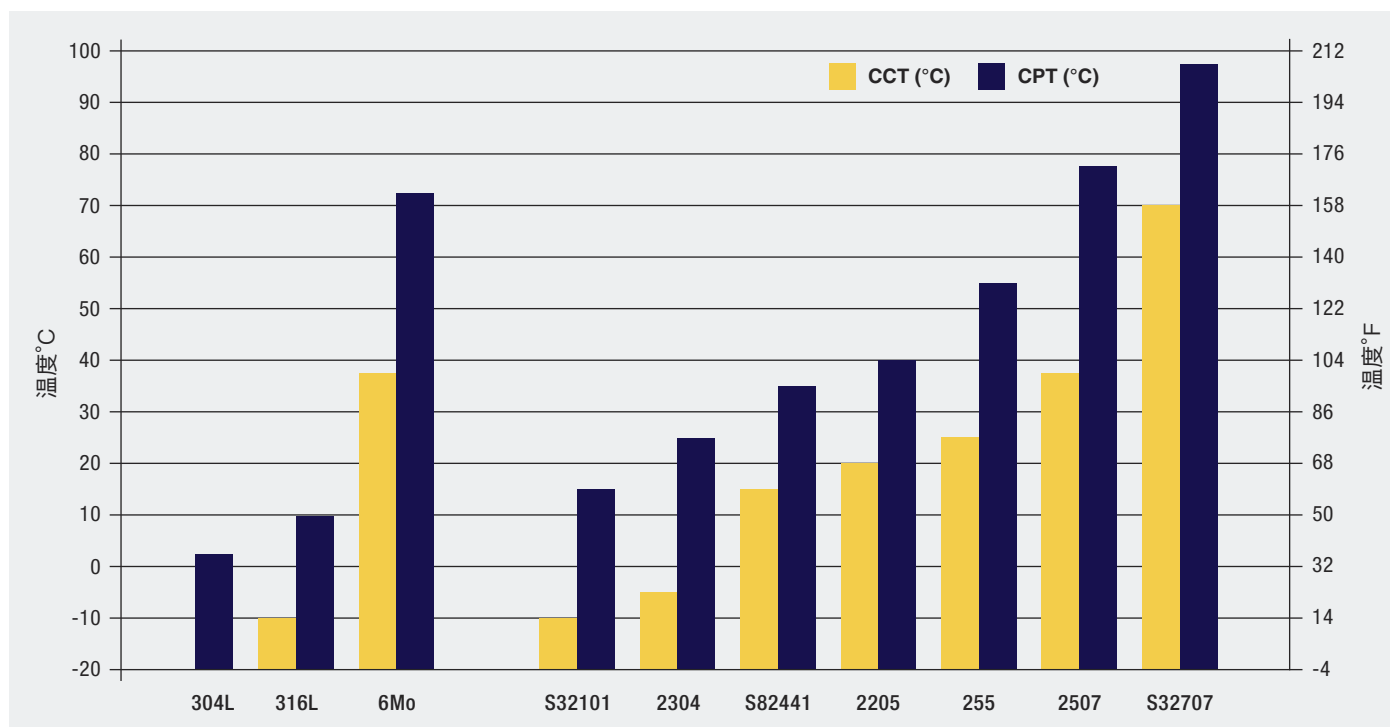
图9 非焊接态奥氏体不锈钢（左）和固溶退火的双相不锈钢（右）的临界点蚀和缝隙腐蚀温度（按照ASTM G48 在6%的三氯化铁溶液中测量）
