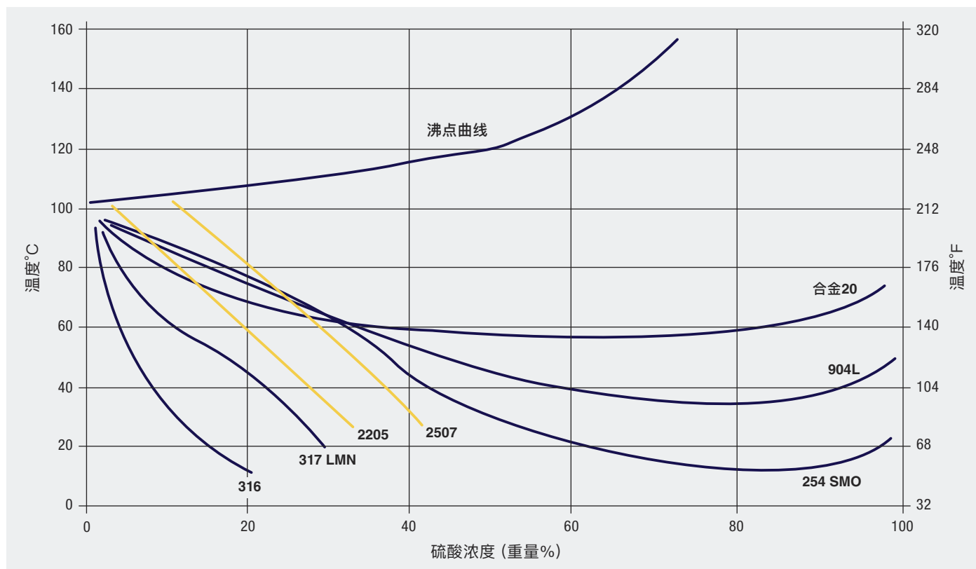
图7 在不含氧的硫酸中的腐蚀，0.1毫米/年 (0.004英寸/年) 等腐蚀曲线 (实验室采用试剂纯度的硫酸) (来源：生产商家材料单，254SMO是Outokumpu的商标)
