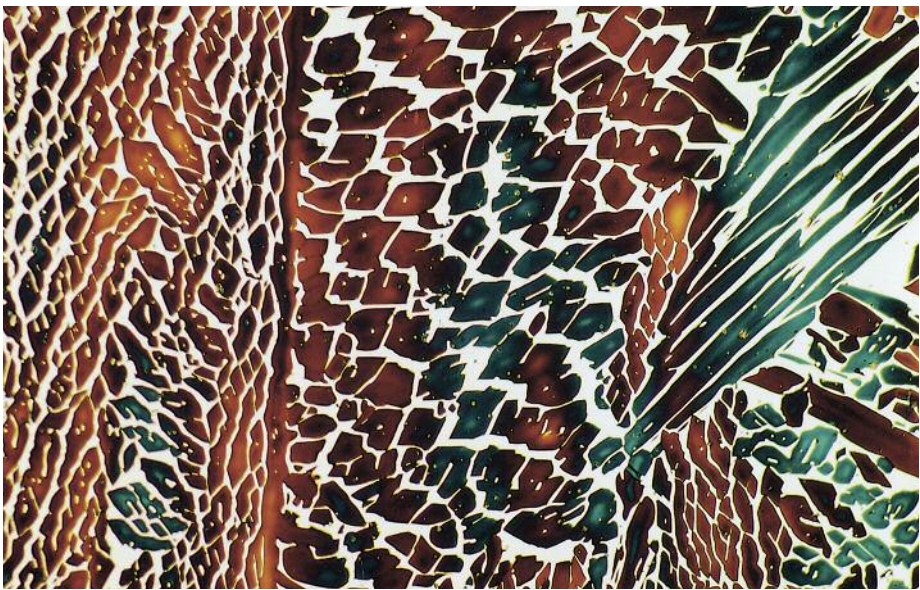
2205双相钢焊缝金属的金相组织，500× © Lincoln Smitweld bv
