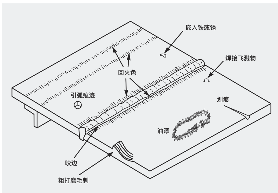
图19 常见加工缺陷或表面状况 (来源：镍协会出版物10026)
