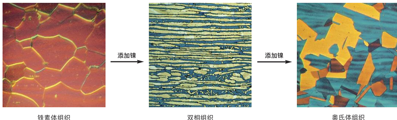
图2 增加镍含量使不锈钢的显微组织从铁素体（左）转变为双相（中）直至奥氏体（右）（这些照片由Outokumpu提供，显示了光学显微镜下放大的经抛光和侵蚀试样的组织。双相组织中，铁素体被染色，呈深色）
