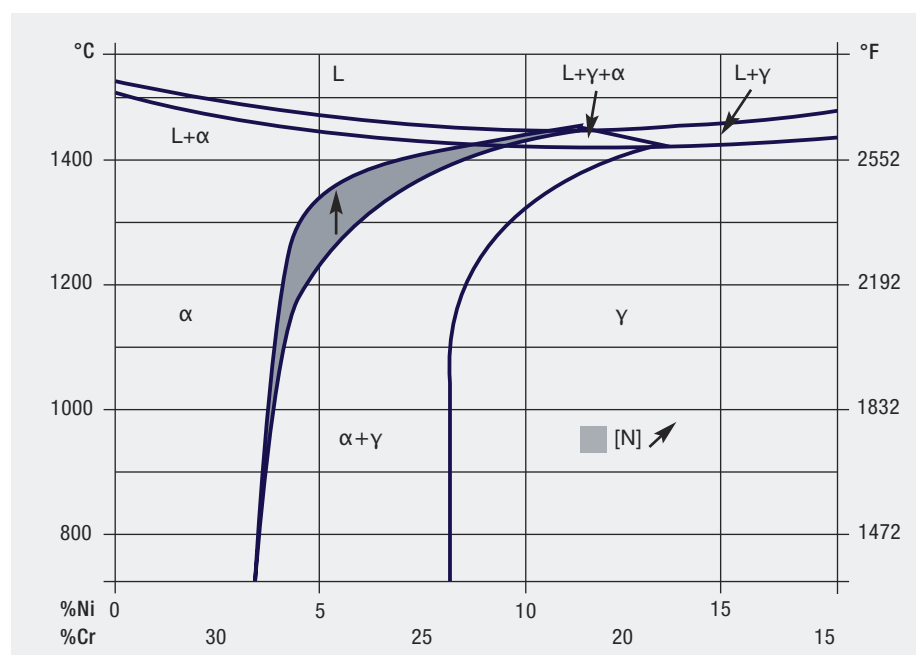
图3 Fe-Cr-Ni三元相图的68%Fe截面图(镍和铬含量微小的变化对双相不锈钢中奥氏体和铁素体的数量有很大的影响)
