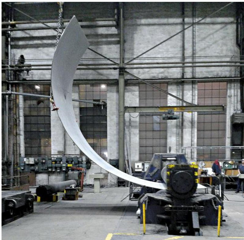
28mm厚双相不锈钢板的卷板机弯曲成形 © Outokumpu
