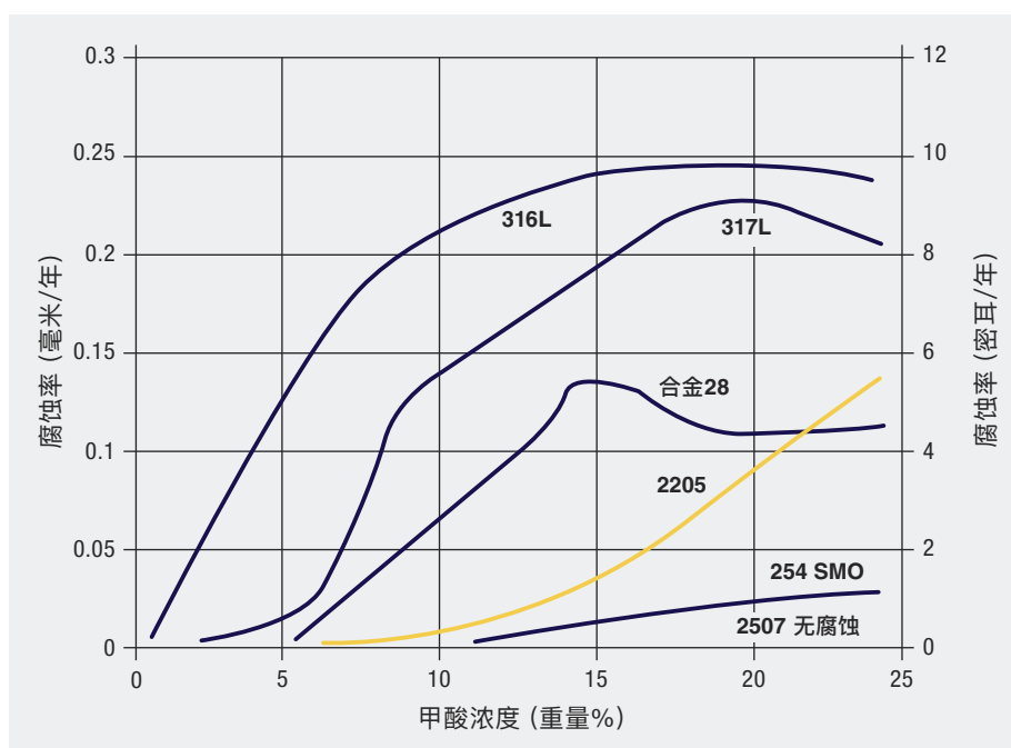
图8 双相不锈钢和奥氏体不锈钢在50%醋酸和不同含量甲酸的沸腾混合溶液中的腐蚀 (来源：Sandvik)
