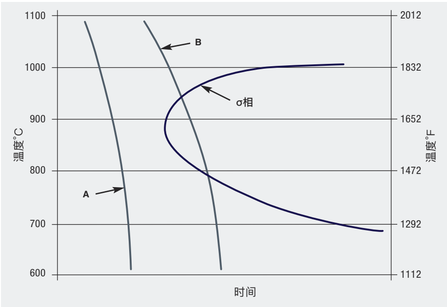
图6 从固溶退火温度冷却应该足够快 (冷却曲线A) 以避免σ相的形成区间 (冷却曲线B)
