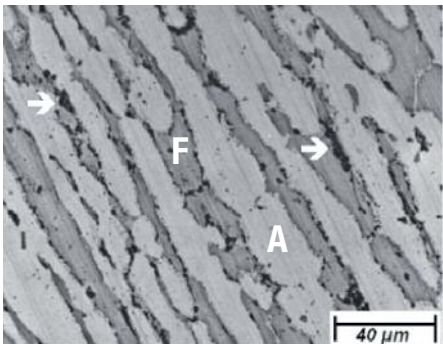
图5 在850°C (1560°F) 下时效处理40分钟的2205样品的显微组织，显示了在奥氏体/铁素体晶界析出的σ相 (箭头)。照片中铁素体相 (F) 比奥氏体相 (A) 颜色深 [3]
