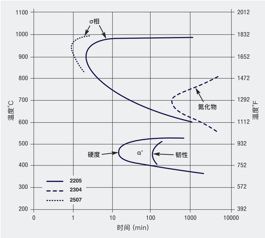
图4 2205双相不锈钢等温析出曲线，1050°C (1920°F) 退火 (分别给出了2304和2507双相钢σ相和氮化物析出曲线作为对比)
