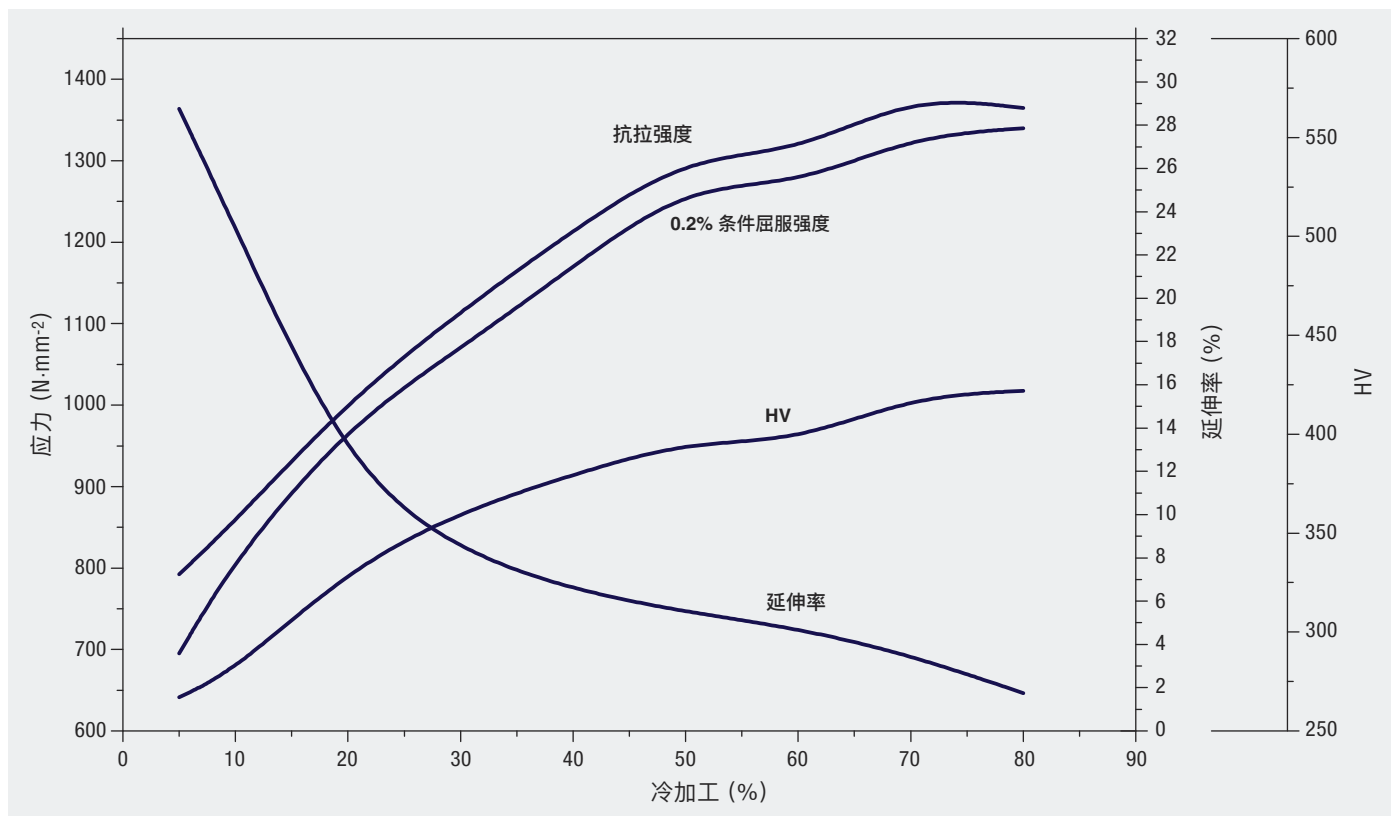
图14 冷加工对2205双相不锈钢力学性能的影响 (来源: 宝钢)
