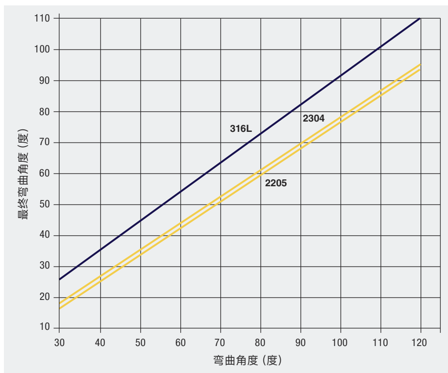
图13 2毫米 (0.08英寸) 厚的双相不锈钢板与316L奥氏体不锈钢板回弹的比较 (来源: Outokumpu)
