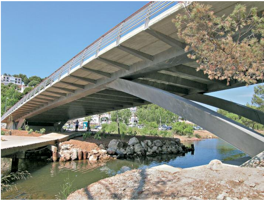
西班牙梅诺卡Cala Galdana 桥采用双相不锈钢2205建造 © PEDELTA
