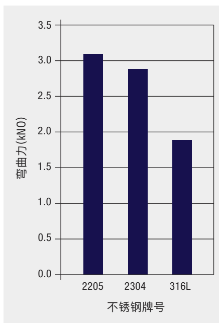
图15 2304, 2205和316L不锈钢弯曲过程中开始塑性变形所需的最小外力，试样宽50毫米(2英寸)，厚2毫米(0.08英寸) (来源: Outokumpu)
