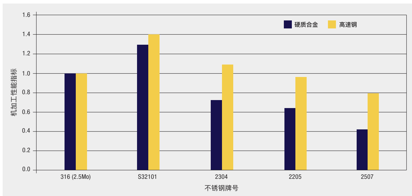
图16 采用硬质合金刀具和高速钢刀具，双相不锈钢和316不锈钢 (2.5Mo) 机加工性能的比较 (来源: Outokumpu)
