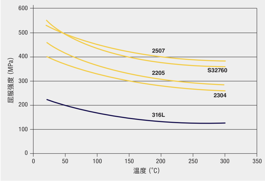
图12 双相不锈钢与316L奥氏体不锈钢在室温到300℃ (572°F) 温度范围典型屈服强度的对比 (来源：生产商数据表)
