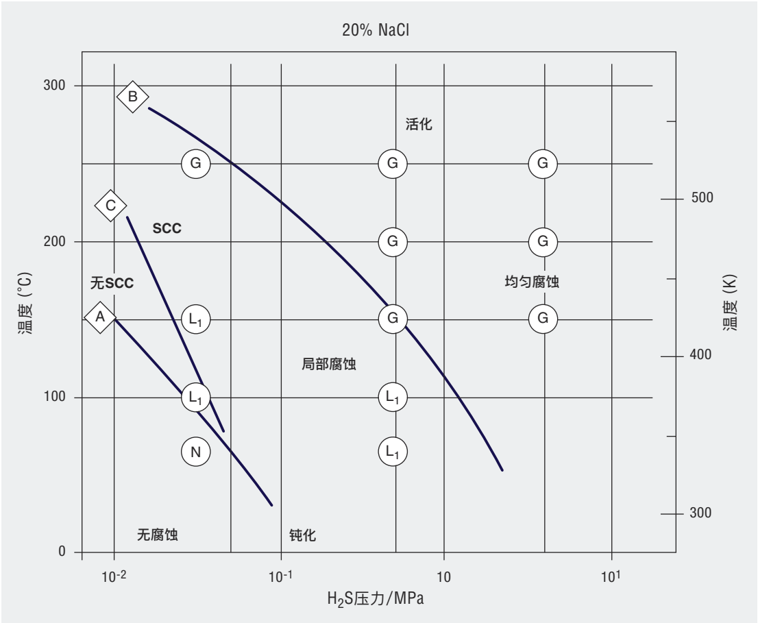
图11 2205双相不锈钢在20%NaCl-H 2 S介质中腐蚀的电化学预测和实验结果
