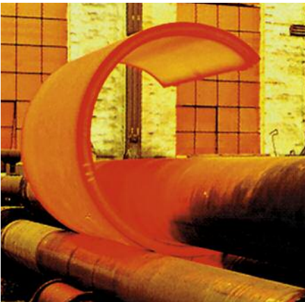
双相不锈钢板的热轧辊弯曲操作 © Outokumpu
