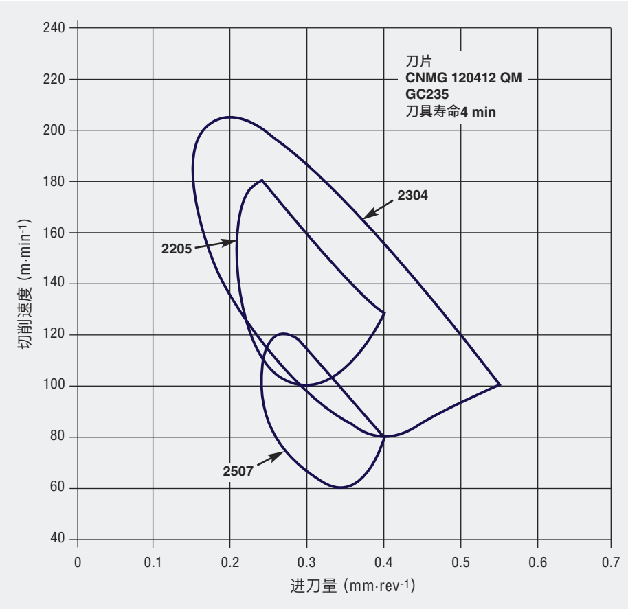
图17 采用硬质合金刀具车削双相不锈钢车削参数的比较，刀具寿命为4分钟 (来源：Sandvik)
