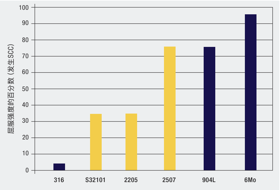
图10 轧制退火的双相不锈钢和奥氏体不锈钢在120℃ (248°F) 氯化钠溶液液滴蒸发试验中的耐应力腐蚀断裂性能（造成断裂的应力以屈服强度的百分数表示） (来源：Outokumpu)
