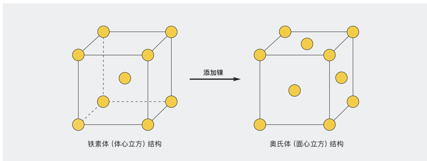
图1 通过添加镍，使晶体结构从体心立方结构（很少量的镍或无镍）转变为面心立方结构（至少6%的镍 – 300系）。含有中等镍含量的双相不锈钢组织中一些晶粒是铁素体，一些晶粒是奥氏体，其理想状态是二者数量相等（图2）
